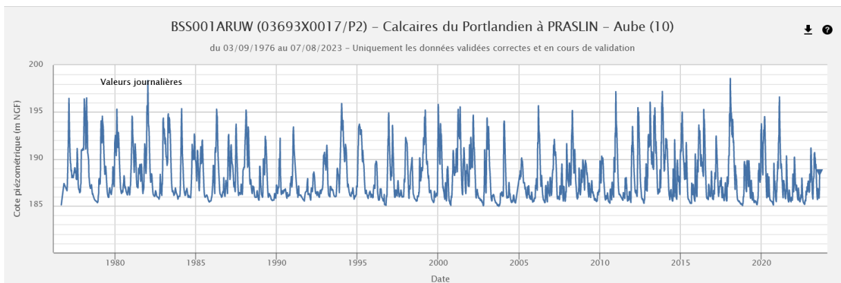
Chronique piézométrique (1976-2023) de Praslin (10), extraction ADES du 07/08/2023
