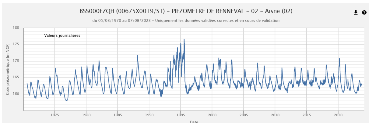
Chronique piézométrique (1970-2023) de Renneval (02), extraction ADES du 07/08/2023
