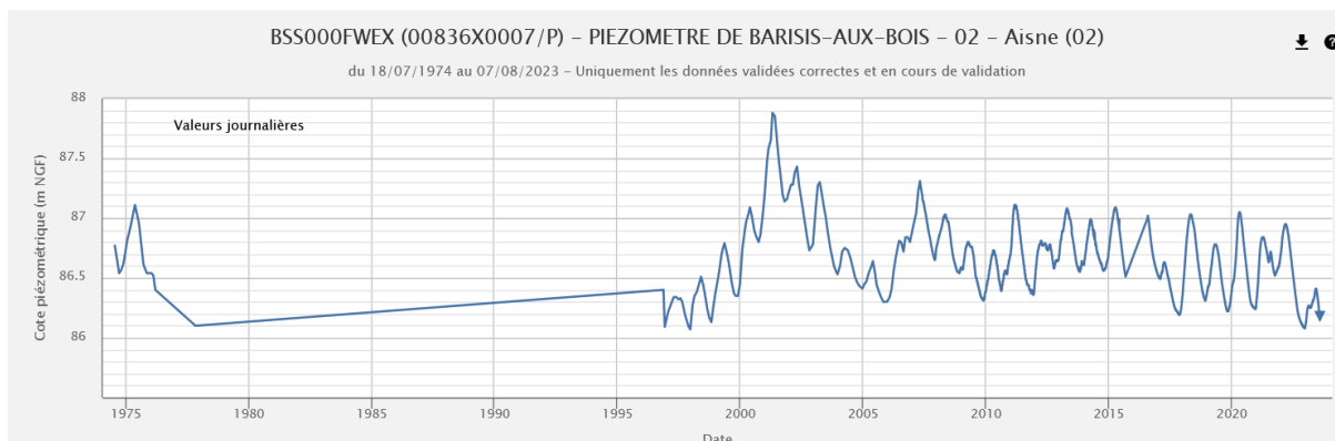
Chronique piézométrique (1974-2023) de Barisis-aux-Bois (02), extraction ADES du 07/08/2023
