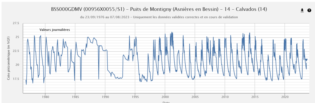
Chronique piézométrique (1976-2023) d'Asnières-en-Bessin (14), extraction ADES du 07/08/2023
