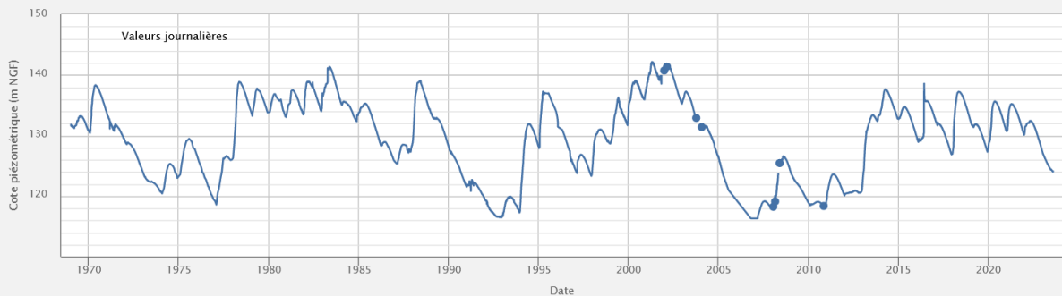
Chronique piézométrique (1969-2023) de Saint-Martin-Chennetron (77), extraction ADES du 07/08/2023
