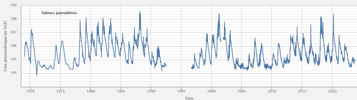
Chronique piézométrique (1969-2023) de Mécringes (51), extraction ADES du 07/08/2023
