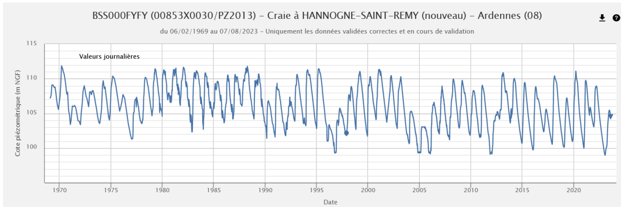
Chronique piézométrique (1969-2023) de Hannogne-Saint-Remy (08), extraction ADES du 07/08/2023
