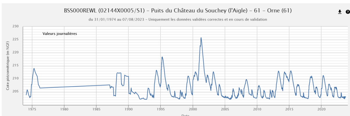
Chronique piézométrique (1971-2023) de Saint-Sulpice-sur-Risle (61), extraction ADES du 07/08/2023
