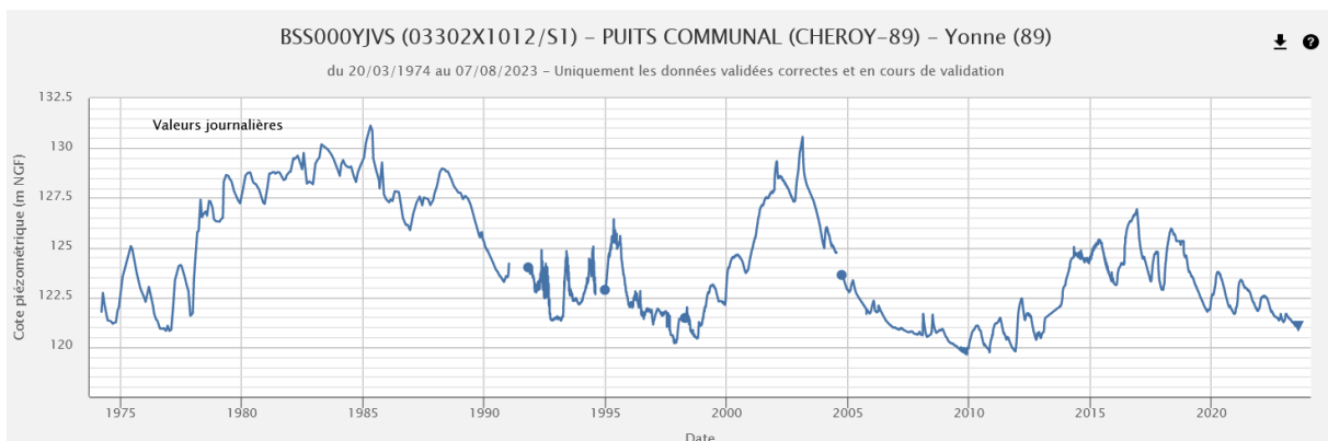
Chronique piézométrique (1974-2023) de Chéroy (89), extraction ADES du 07/08/2023
