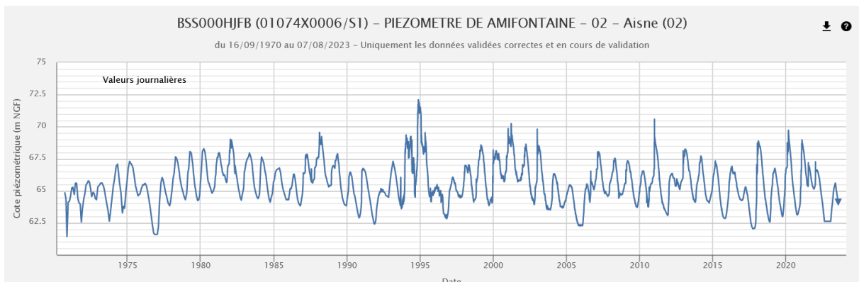
Chronique piézométrique (1970-2023) d'Amifontaine (02), extraction ADES du 07/08/2023
