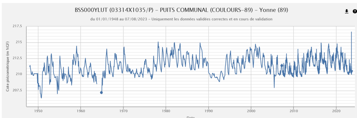
Chronique piézométrique (1948-2023) de Couleurs (89), extraction ADES du 07/08/2023
