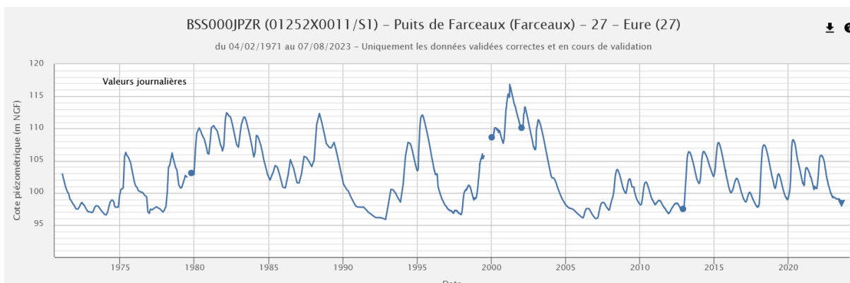
Chronique piézométrique (1971-2023) de Farceaux (27), extraction ADES du 07/08/2023
