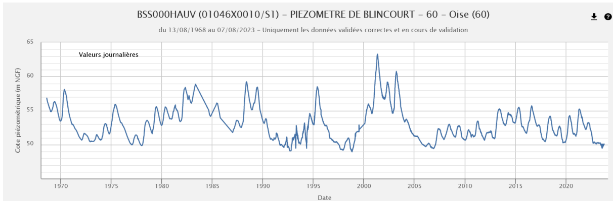
Chronique piézométrique (1968-2023) de Blincourt (60), extraction ADES du 07/08/2023
