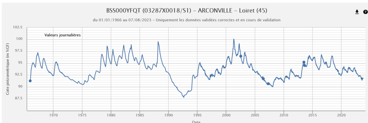
Chronique piézométrique (1966-2023) de Batilly-en-Gâtinais (45), extraction ADES du 07/08/2023
