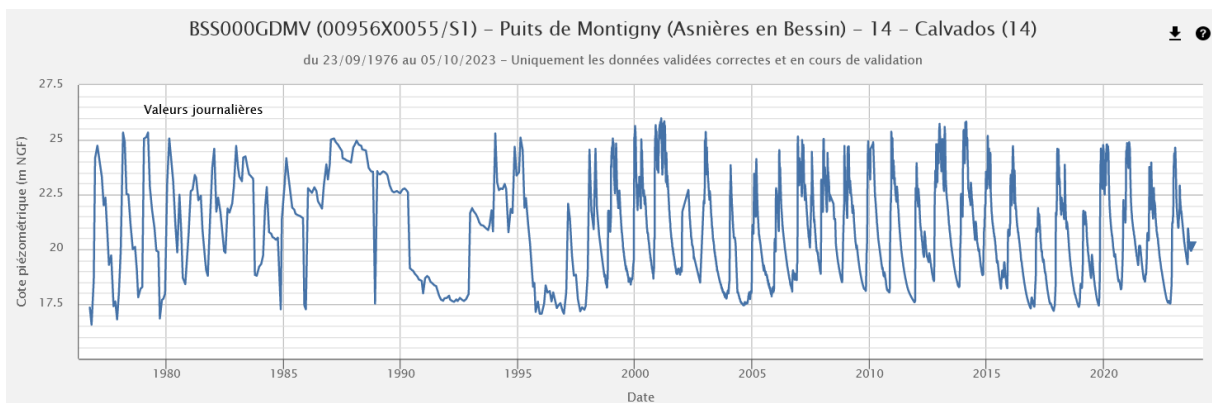
Chronique piézométrique (1976-2023) d'Asnières-en-Bessin (14), extraction ADES du 05/10/2023
