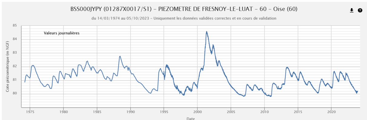
Chronique piézométrique (1974-2023) de Fresnoy-le-Luat (60), extraction ADES du 05/10/2023
