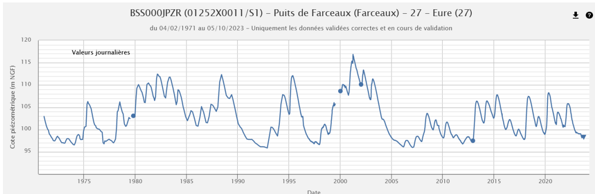
Chronique piézométrique (1971-2023) de Farceaux (27), extraction ADES du 05/10/2023
