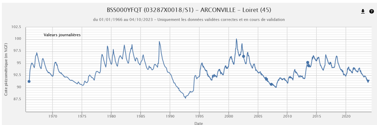
Chronique piézométrique (1966-2023) de Batilly-en-Gâtinais (45), extraction ADES du 05/10/2023
