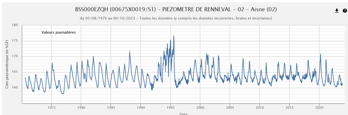
Chronique piézométrique (1970-2023) de Renneval (02), extraction ADES du 04/10/2023
