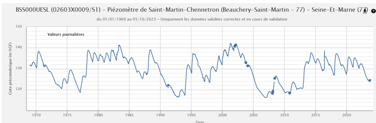
Chronique piézométrique (1969-2023) de Saint-Martin-Chennetron (77), extraction ADES du 05/10/2023
