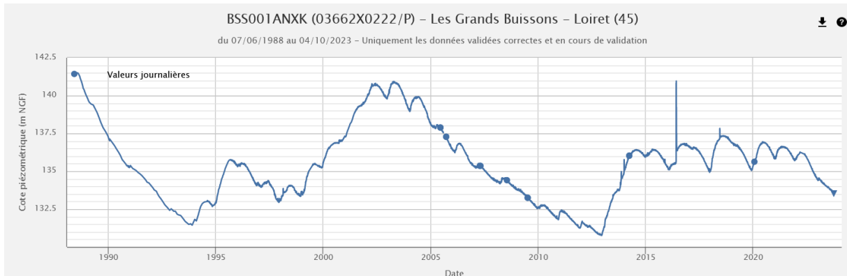
Chronique piézométrique (1988-2023) de Chuelles (45), extraction ADES du 05/10/2023
