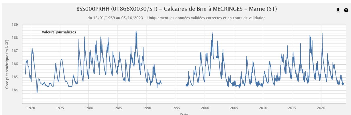
Chronique piézométrique (1969-2023) de Mécringes (51), extraction ADES du 05/10/2023
