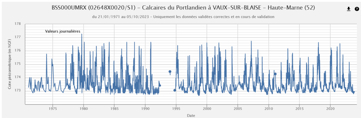
Chronique piézométrique (1971-2023) de Vaux-sur-Blaise (52), extraction ADES du 05/10/2023
