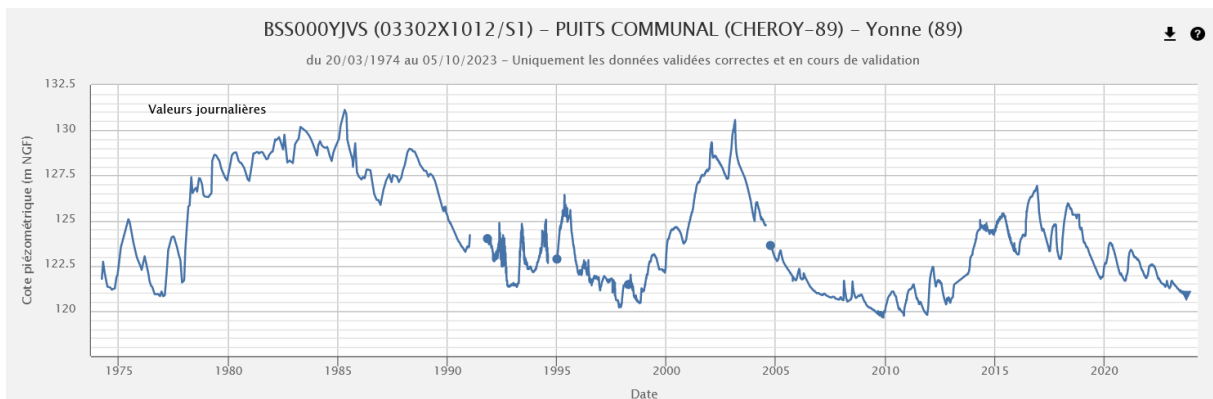
Chronique piézométrique (1974-2023) de Cheroy (89), extraction ADES du 05/10/2023
