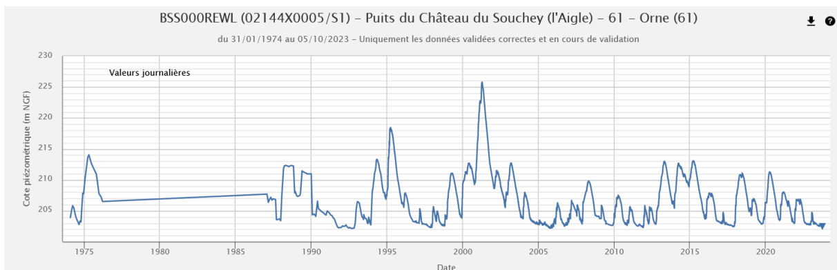
Chronique piézométrique (1971-2023) de Saint-Sulpice-sur-Risle (61), extraction ADES du 05/10/2023
