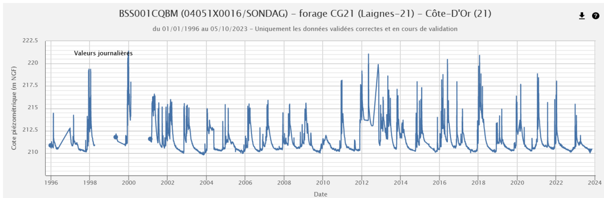
Chronique piézométrique (1996-2023) de Laignes (21), extraction ADES du 05/10/2023
