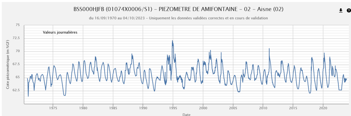
Chronique piézométrique (1970-2023) d'Amifontaine (02), extraction ADES du 04/10/2023
