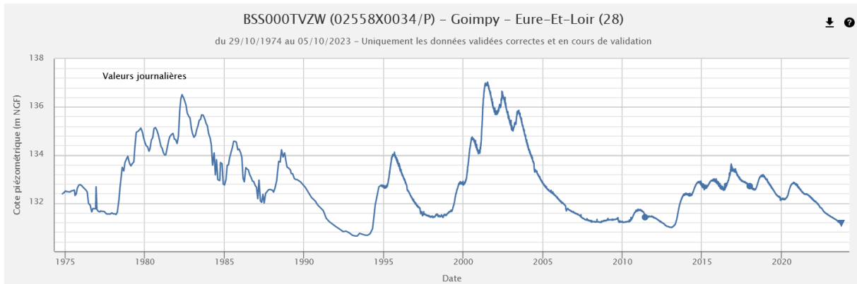
Chronique piézométrique (1974-2023) de Saint-Léger-les-Aubées (28), extraction ADES du 05/10/2023
