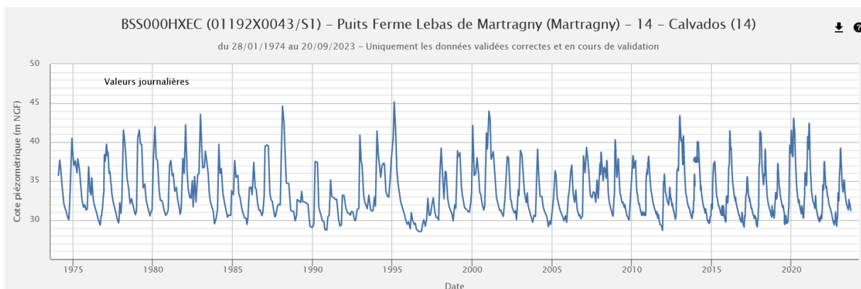
Chronique piézométrique (1974-2023) de Martragny (14), extraction ADES du 05/10/2023
