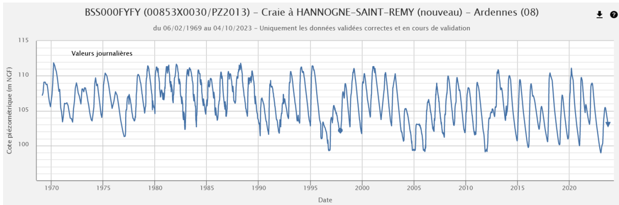
Chronique piézométrique (1969-2023) de Hannogne-Saint-Remy (08), extraction ADES du 04/10/2023
