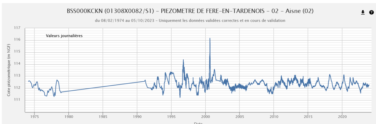
Chronique piézométrique (1974-2023) de Fère-en-Tardenois (02), extraction ADES du 05/10/2023
