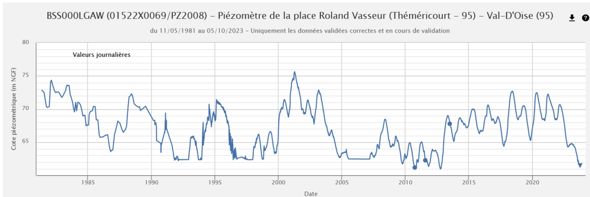
Chronique piézométrique (1981-2023) de Théméricourt (95), extraction ADES du 05/10/2023
