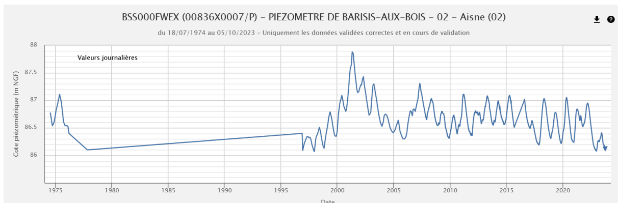
Chronique piézométrique (1974-2023) de Barisis-aux-Bois (02), extraction ADES du 05/10/2023
