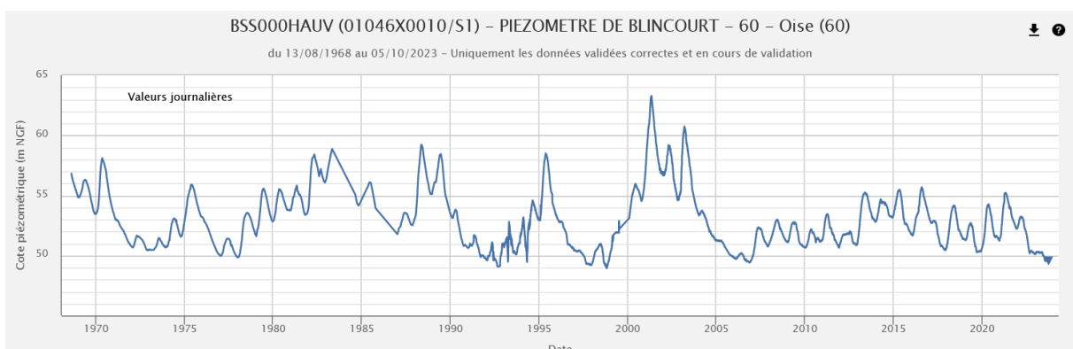
Chronique piézométrique (1968-2023) de Blincourt (60), extraction ADES du 05/10/2023
