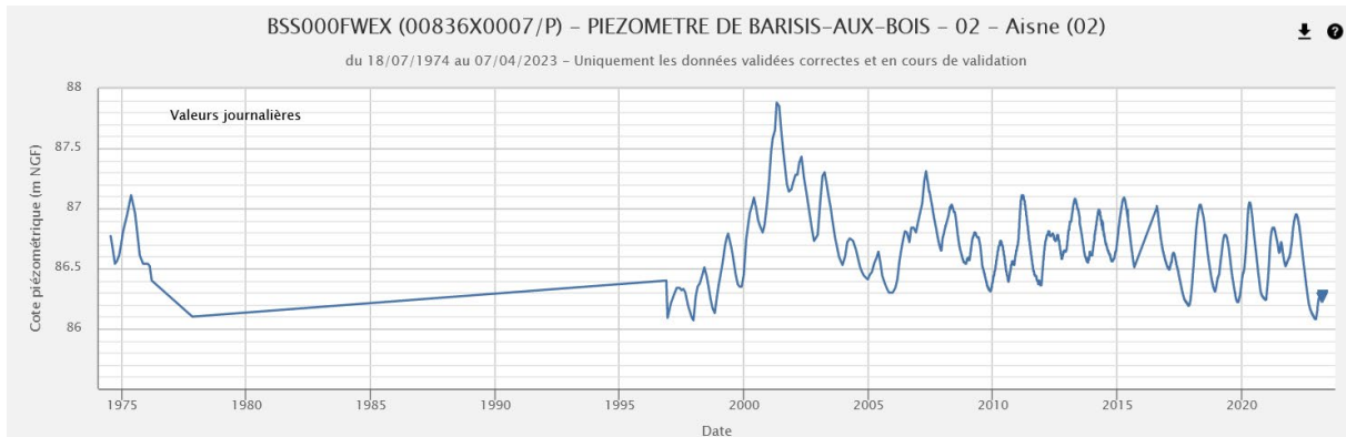
Chronique piézométrique (1974-2023) de Barisis-aux-Bois (02), extraction ADES du 07/04/2023
