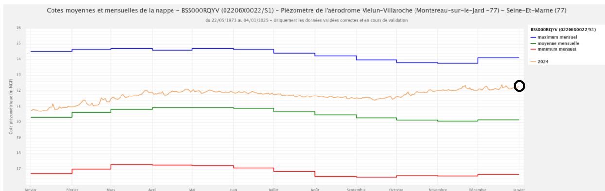
Figure 8. Chronique piézométrique (2024) de Montereau-sur-le-Jard (77), extraction ADES du 07/01/2025.
