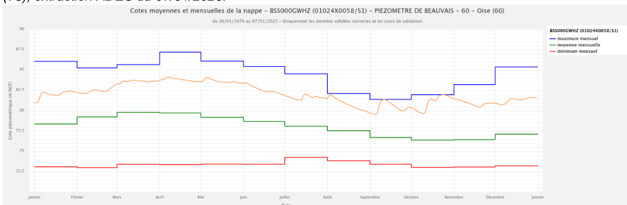
Figure 13. Chronique piézométrique (2024) de Beauvais (60), extraction ADES du 07/01/2025.
