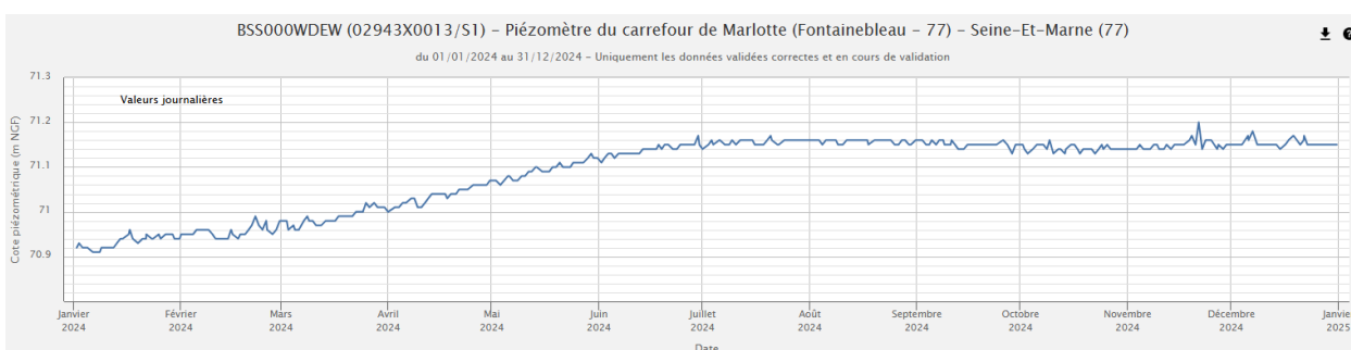
Figure 3. Chronique piézométrique 2024 de Fontainebleau (77), extraction ADES du 07/01/2025.
