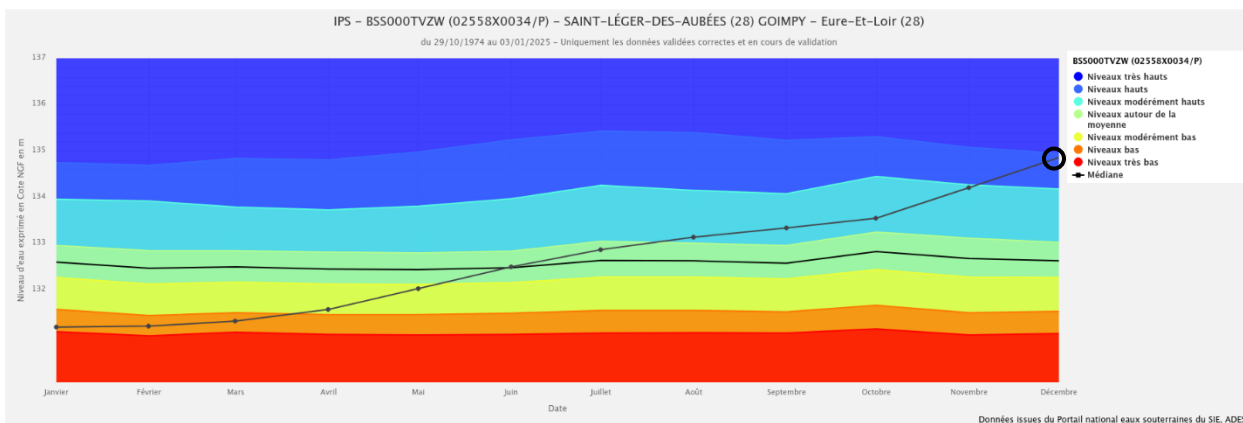
Figure 5. Évolution de l'IPS en 2024 à Saint-Léger-des-Aubées (28), extraction ADES du 07/01/2025.
