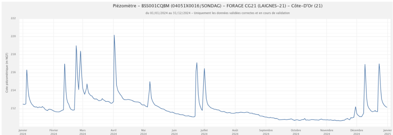
Figure 22. Chronique piézométrique (2024) de Laignes (89), extraction ADES du 07/01/2024.
