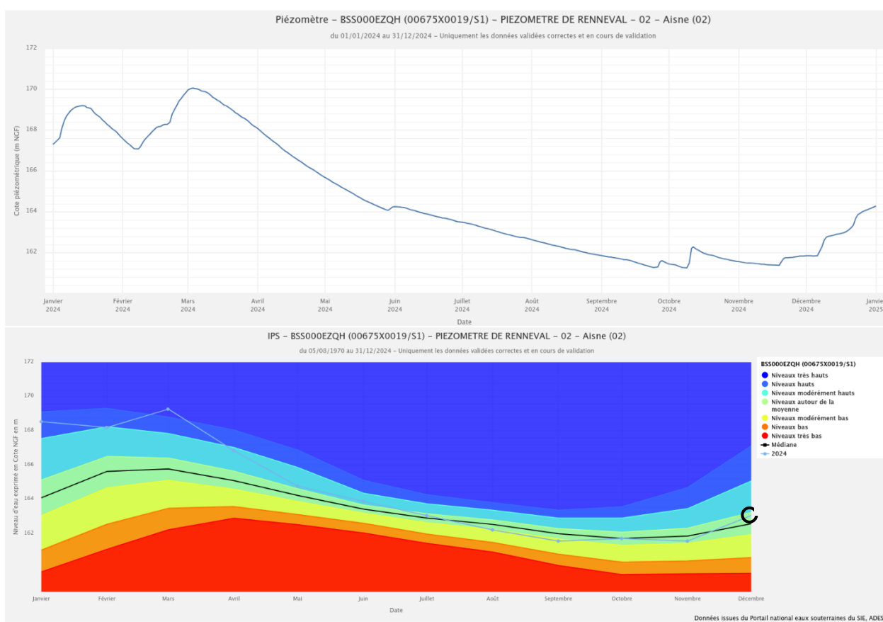
Figure 16. Chronique piézométrique (2024) et évolution de l'IPS en 2024 du piézomètre de Renneval (02), extraction ADES du 07/01/2025.
