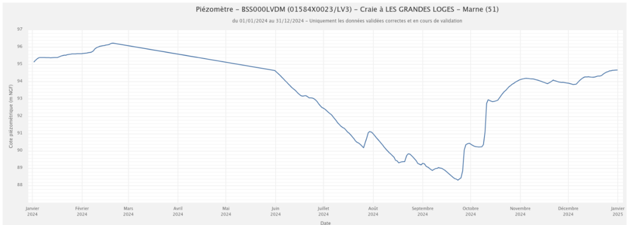
Figure 17. Chronique piézométrique (2024) du piézomètre Les Grands Loges (51), extraction ADES du 07/01/2025.
