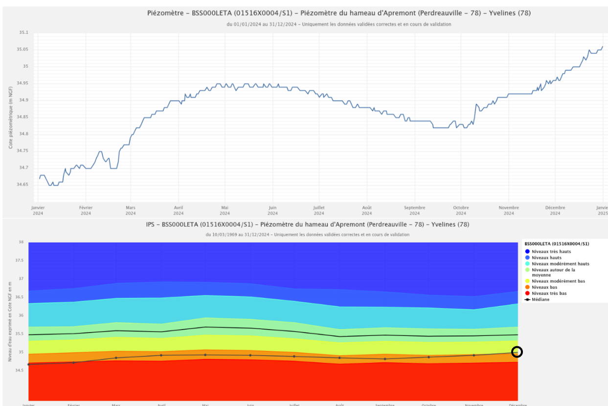
Figure 12. Chronique piézométrique (2024) et évolution de l'IPS en 2024 du piézomètre de Perdreauville (78), extraction ADES du 07/01/2025.
