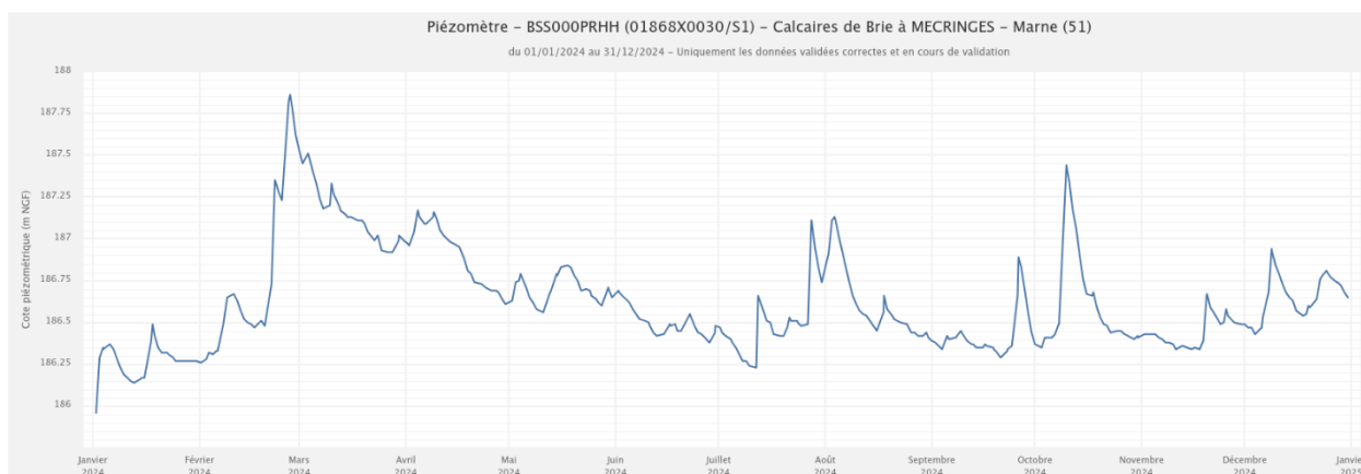
Figure 6. Chronique piézométrique 2024 de Mécringes (51), extraction ADES du 07/01/2025.
