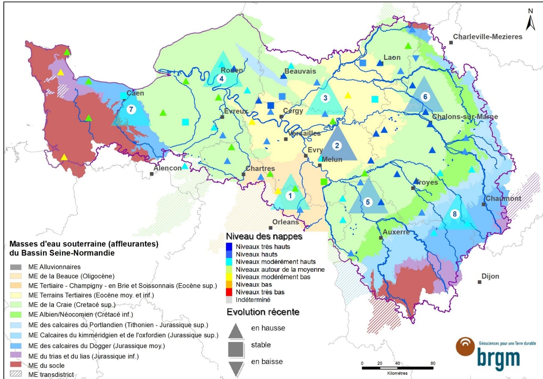
Figure 2. Carte du niveau des nappes du bassin Seine-Normandie et leur évolution récente (mis à jour le 08/01/2025)
