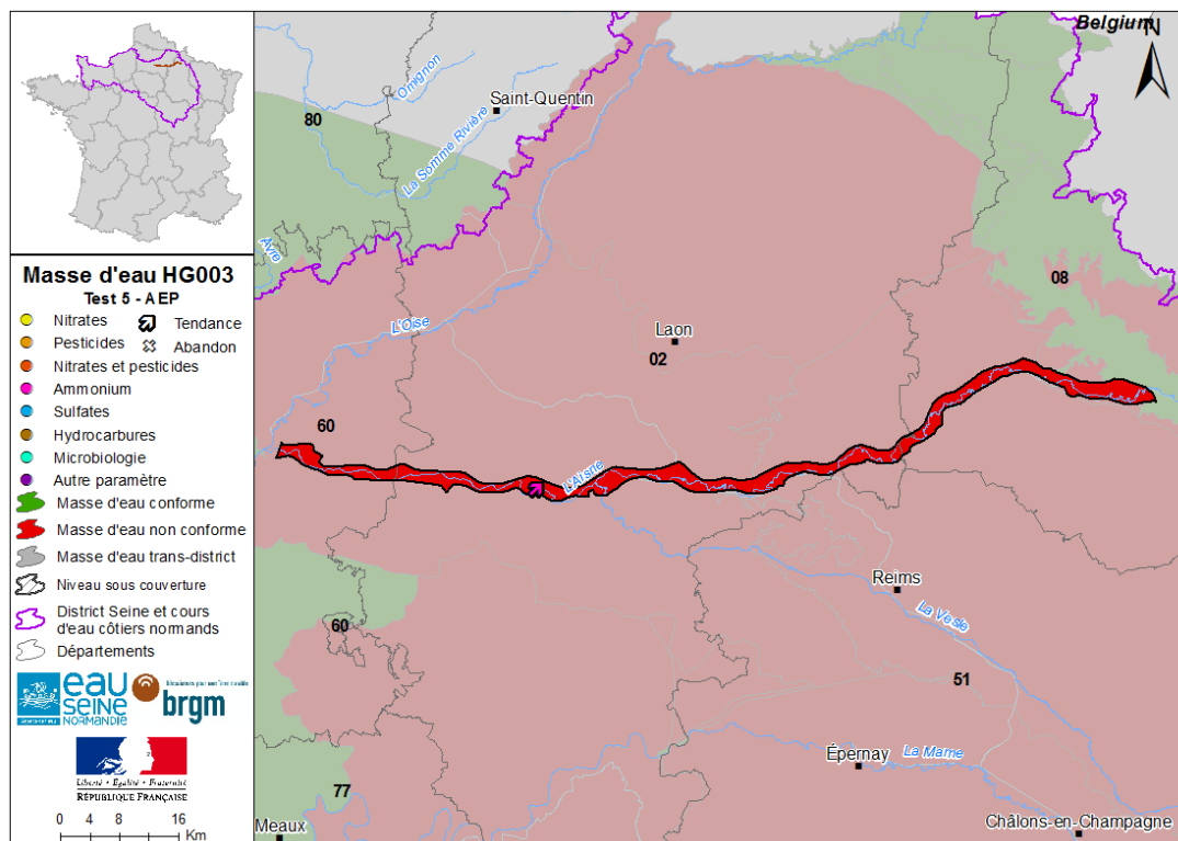
Figure 3 : Carte du test 5 « zone protégée pour l'Alimentation en Eau Potable » de la masse d'eau souterraine HG003 (tendances à la hausse avec dépassement des normes/valeurs-seuils des points AEP et abandon des captages pour cause de qualité). Source : AESN, ARS, ADES.
