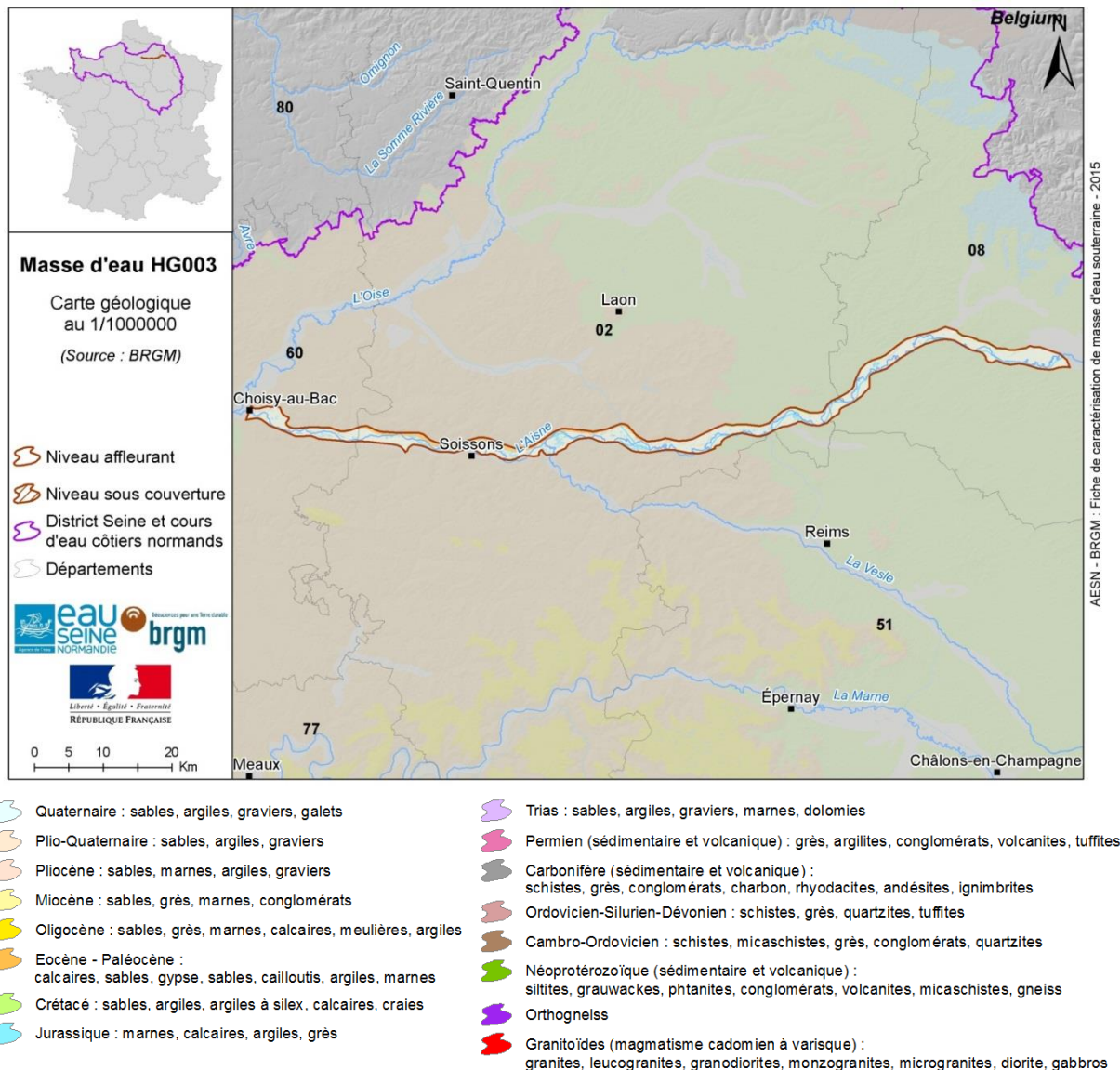
Figure 1 : Carte géologique de la masse d'eau souterraine HG003. Source : BRGM.
