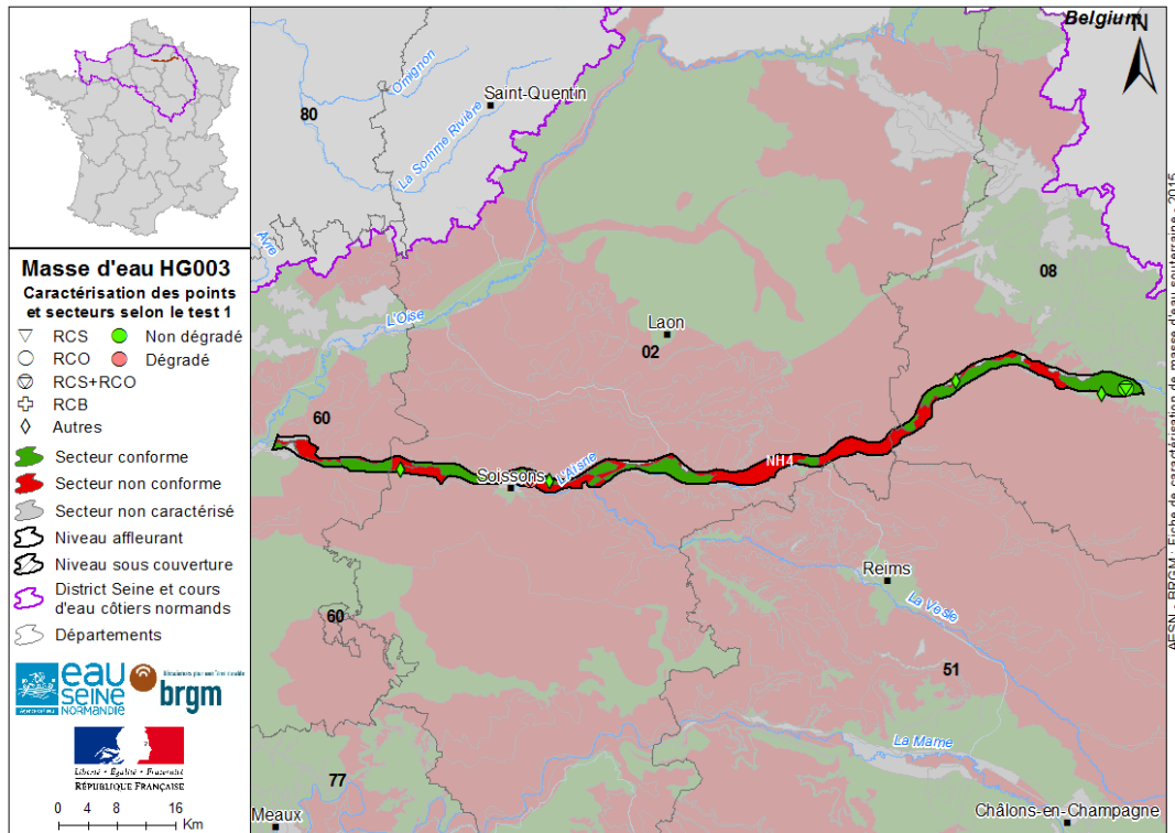
Figure 2 : Carte du test 1 « qualité générale » de la masse d'eau souterraine HG003 (surfaces concernées par le dépassement des normes / valeurs-seuils ou fréquences de dépassement > 20%). Source : AESN, ARS, ADES.
