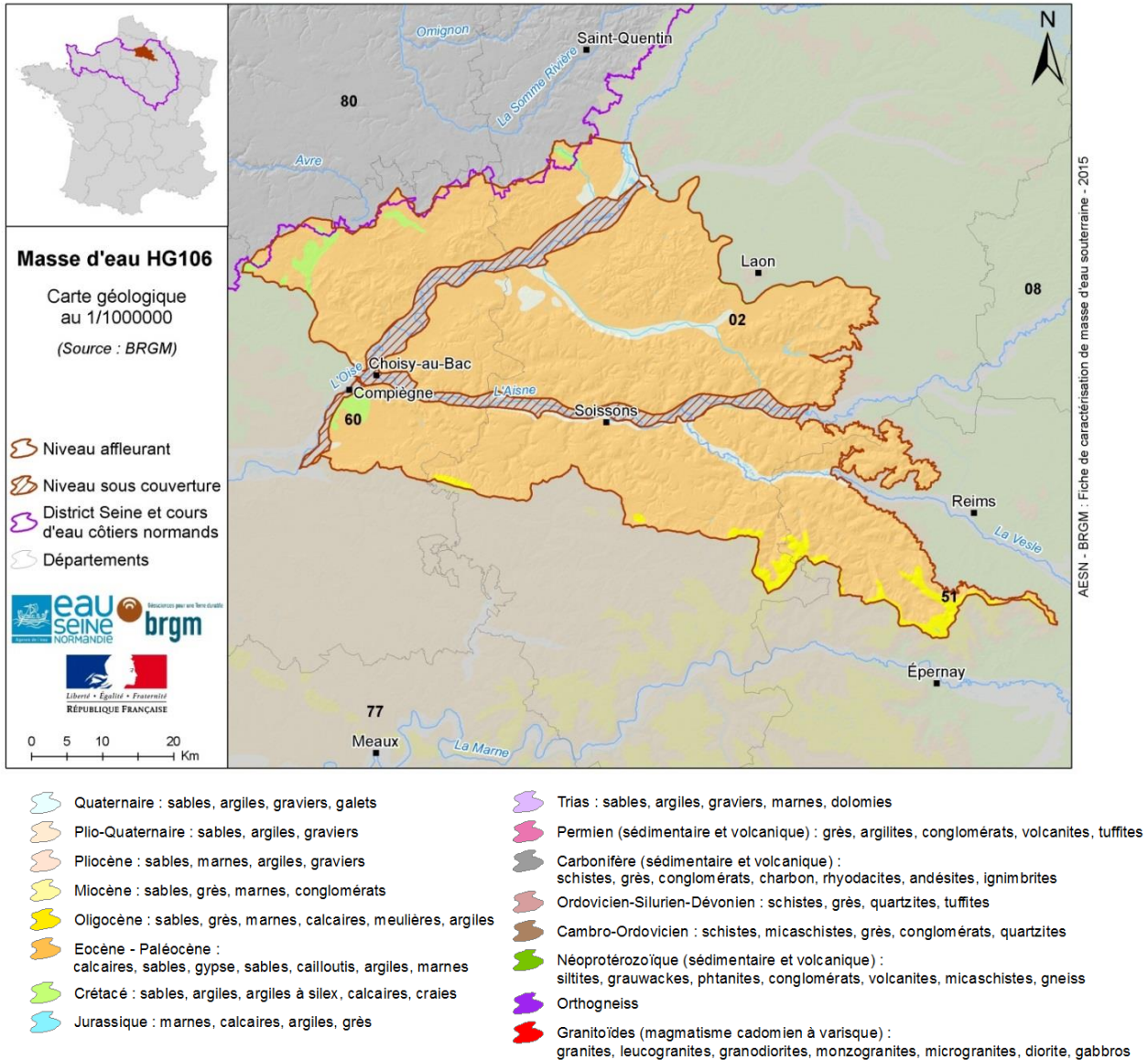
Figure 1 : Carte géologique de la masse d'eau souterraine HG106. Source : BRGM.
