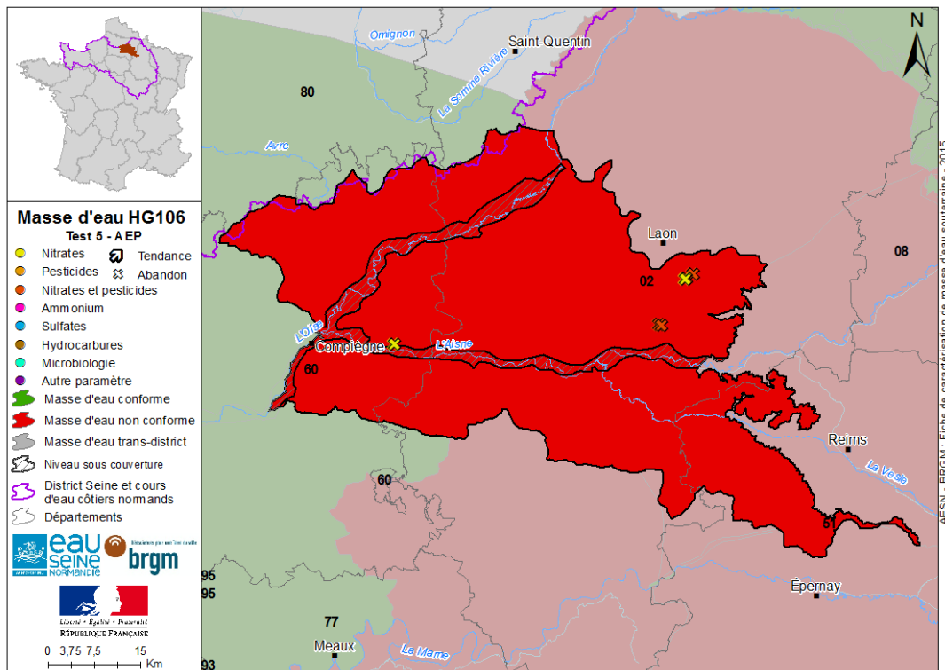
Figure 3 : Carte du test 5 « zone protégée pour l'Alimentation en Eau Potable » de la masse d'eau souterraine HG106 (tendances à la hausse avec dépassement des normes/valeurs-seuils des points AEP et abandon des captages pour cause de qualité). Source : AESN, ARS, ADES.
