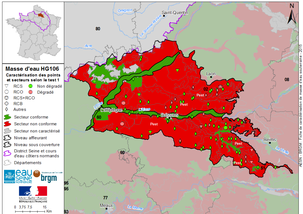
Figure 2 : Carte du test 1 « qualité générale » de la masse d'eau souterraine HG106 (surfaces concernées par le dépassement des normes / valeurs-seuils ou fréquences de dépassement > 20%). Source : AESN, ARS, ADES.
