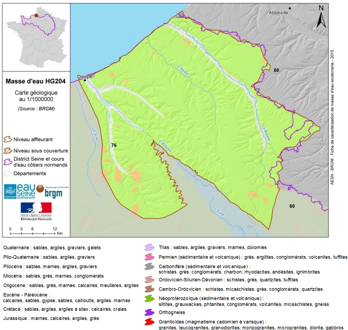
Figure 1 : Carte géologique de la masse d'eau souterraine HG204. Source : BRGM.
