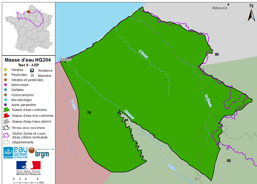
Figure 3 : Carte du test 5 « zone protégée pour l'Alimentation en Eau Potable » de la masse d'eau souterraine HG204 (tendances à la hausse avec dépassement des normes/valeurs-seuils des points AEP et abandon des captages pour cause de qualité). Source : AESN, ARS, ADES.
