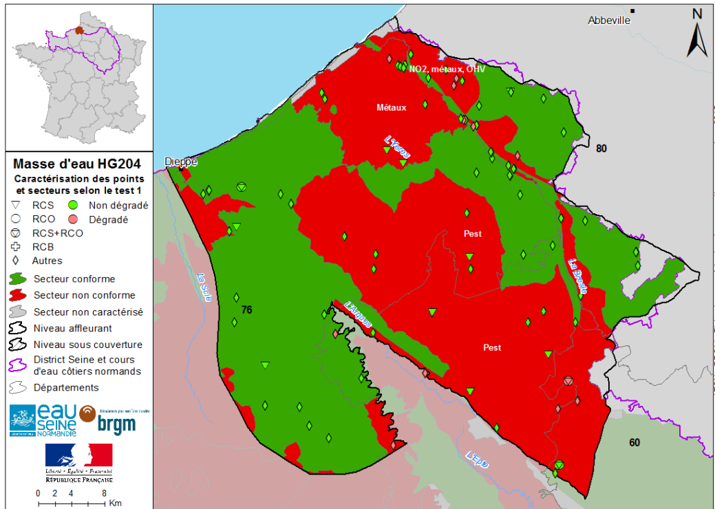
Figure 2 : Carte du test 1 « qualité générale » de la masse d'eau souterraine HG204 (surfaces concernées par le dépassement des normes / valeurs-seuils ou fréquences de dépassement > 20%). Source : AESN, ARS, ADES.
